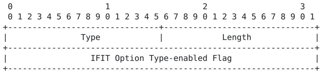
Fig. 1 IFIT Node Capability sub-TLV Format
