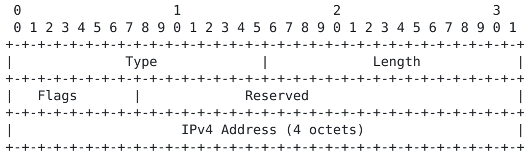
IPv4 ERO Sub-TLV format
