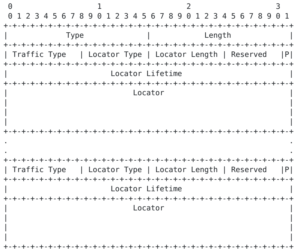
Figure 6: LOCATOR_SET Parameter Format
